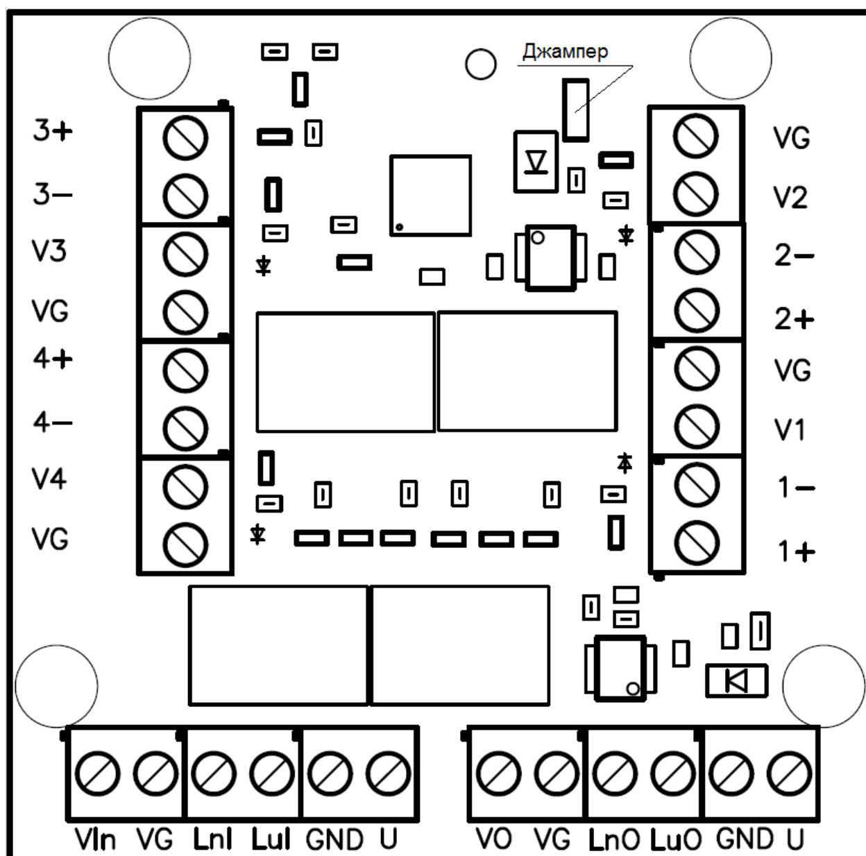
Рис. 2 Вид платы коммутатора этажного комбинированного
