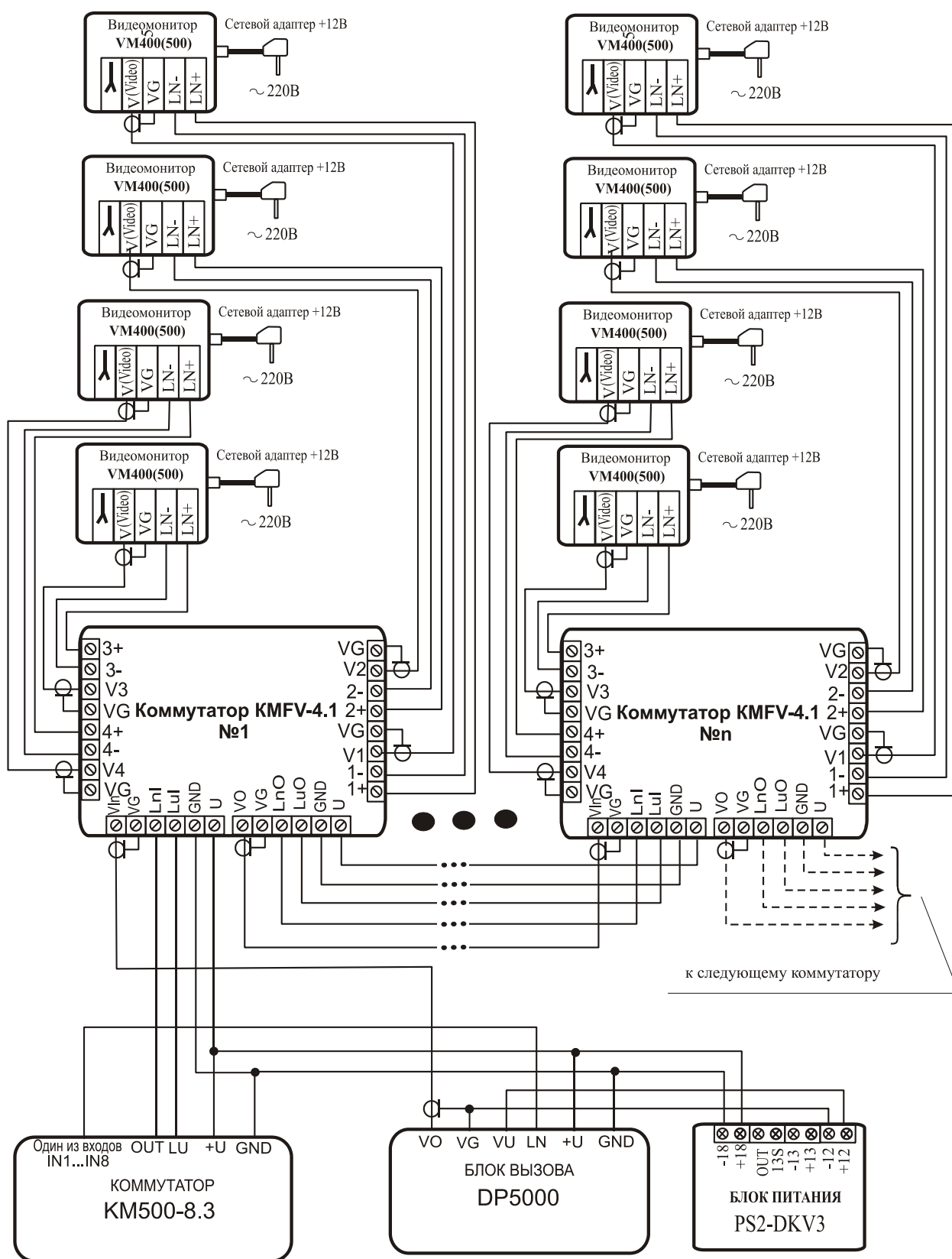
Рис.6 Схема подключения коммутатора этажного KMF- 4.1V в составе сетевого домофонного комплекса ELTIS5000
