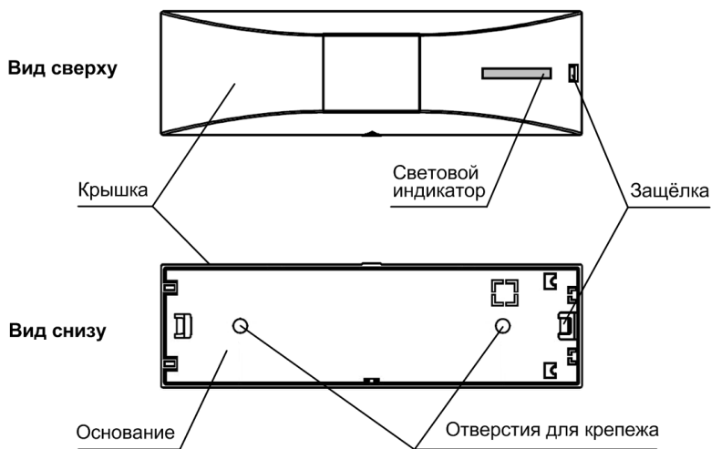
Рис.2 Конструкция сигнализатора. Вид сверху и снизу
