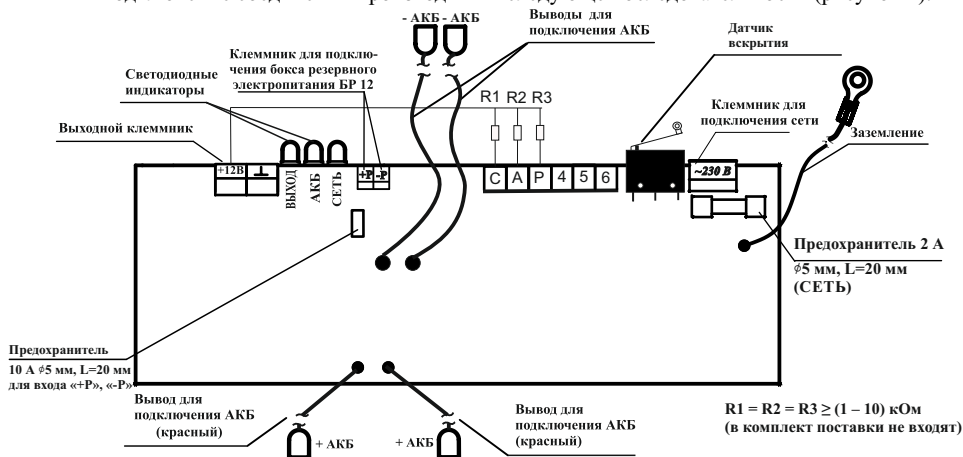
Рисунок 1 – Плата источника
