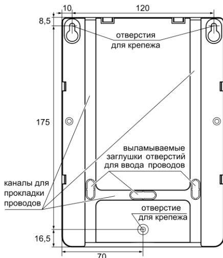
Рис.2 Основание. Присоединительные размеры
