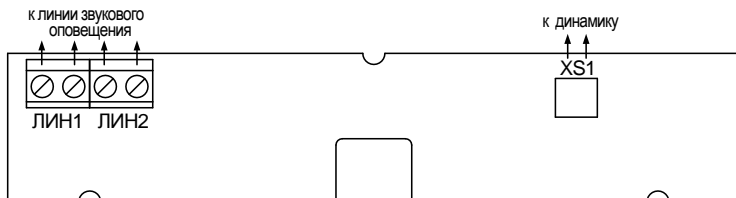
Рис.1 Плата «АС-2-1». Схема соединений
