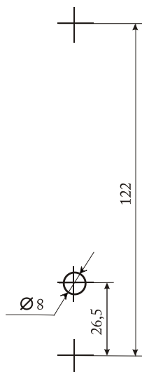
Рис.1. Разметка под установку изделия.
