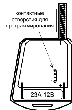
Рис.1. Радиокнопка со снятой задней крышкой
